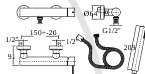
06. Monocomando de base de chuveiro Shower mixer Mitigeur douche avec douchette
