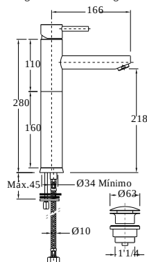
03. Monocomando de lavatório alto Basin mixer for high level washbasin Mitigeur de lavabo allongé avec vidage
