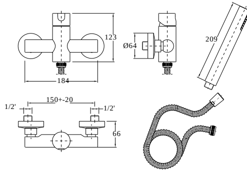
11. Misturadora de banheira de encastrar Wall mounted tap for bathtub Mitigeur Bain/Douche encastré
