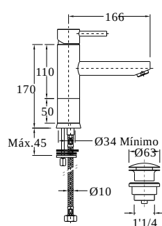
02. Monocomando de lavatório médio Basin mixer Mitigeur de Lavabo moyen avec vidage
