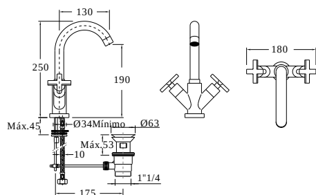
01. Misturadora de lavatório Basin mixer Mitigeur de Lavabo avec vidage
