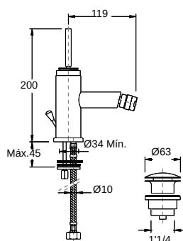
03. Monocomando de bidé Single lever for bidet with pop up Mitigeur de bidet avec vidage click-clack
