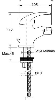
04. Monocomando de bidê Single lever for bidet with pop up Mitigeur bidet avec vidage
