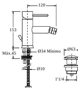
04. Monocomando de bidé Bider mixer Mitigeur de Bidet avec vidage
