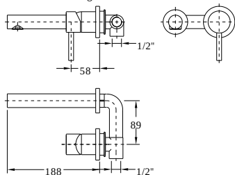
09. Misturadora de lavatório de parede Wall mounted mixer basin Mélangeur 3 trous
