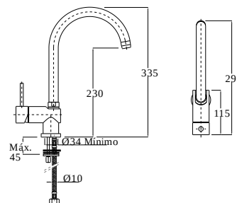
07. Misturadora de banca c/ bica giratória | Kitchen mixer Mitigeur de cuisine avec bec orientable
