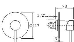
13. Misturadora base de chuveiro encastrar Shower mixer inlay Misturadora base de chuveiro encastrar
