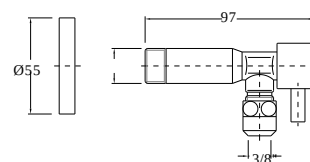
13. Torneira de esquadria Faucet Robinnet d'équerre 1/2 x 3/8
