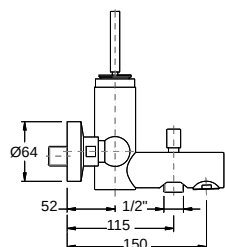
04. Monocomando de banheira Single lever for bathtub Mitigeur de Bain/Douche
