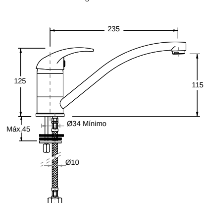
05. Monocomando banca rotativa Kitchen mixer Mitigeur cuisine avec bec orientable
