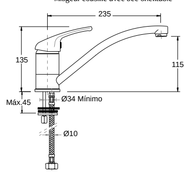
05. Monocomando banca rotativa Kitchen mixer Mitigeur cuisine avec bec orientable
