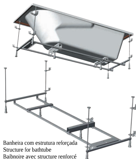
Injector rotativo opcional Rotary jets (optional) Jet rotatif (option)
