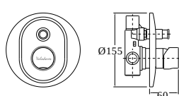
11. Misturadora de banheira de encastrar Wall mounted tap for bathtub Mitigeur Bain/Douche encastré
