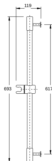
14. Rampa de chuveiro Shower tray Barre Douche
