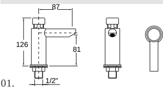
REF. 50649102 01. Torneira temporizada de lavatório Assi 50649112 02. Torneira temporizada de urinol Assi 50649122 03. Torneira temporizada de chuveiro encastrada Assi
