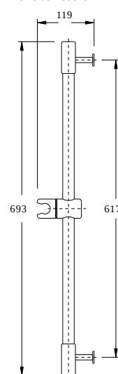
17. Rampa chuveiro | Shower rail Barre de Douche
