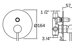
09. Misturadora de base chuveiro de encastrar Wall mounted tap for shower tray Mitigeur douche a encastrar
