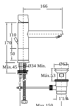
02. Monocomando de lavatório médio Single lever for washbasin medium with pop up Mitigeur de Lavabo sans vidage
