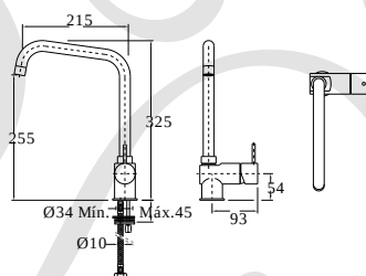
08.Misturadora de banca | Kitchen mixer Mitigeur de cousine
