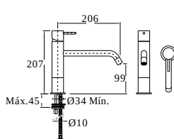
03.Monocomando de lavatório médio Basin mixer Mitigeur de Lavabo moyen avec vidage
