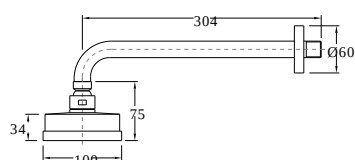
15. Chuveiro c/ haste | Handy shower tray | Tête p/douchete
