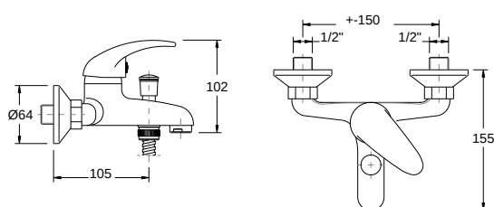
01. Monocomando de banheira Single lever for bathtub Mitigeur de Bain/Douche
