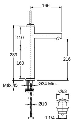
02. Monocomando de lavatório alto Single lever for washbasin high with up Mitigeur de lavabo allongé avec vidage click-clack
