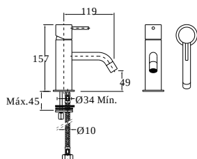
04.Monocomando de bidé Bider mixer Mitigeur de Bidet avec vidage
