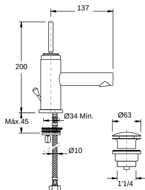
01. Monocomando de lavatório Single lever for washbasin with pop up Mitigeur de lavabo avec vidage click-clack
