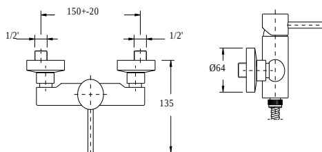
06. Monocomando de base de chuveiro Shower mixer Mitigeur douche avec douchette
