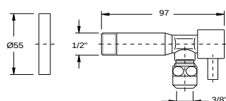
11. Torneira esquadria | Tap 3/8" | Robinet d'equerre 1/2 x 3/8 assi
