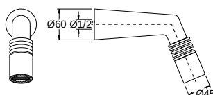
12. Chuveiro c/haste | Arm and rose | Tête douche
