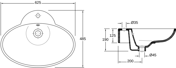
REF. CORES DISPONÍVEIS | AVAILABLE COLOURS | COULEURS DISPONIBLES a) 00 | 16 | 20 b) 01 (VER PÁG. 10 | SEE PAGE 10 | REGARDER PAGE.10) 18701 Miami (62 x 48 cm)
