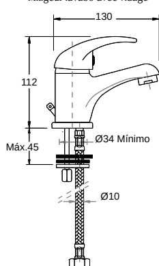
03. Monocomando de lavatório Single lever for washbasin with pop up Mitigeur lavabo avec vidage
